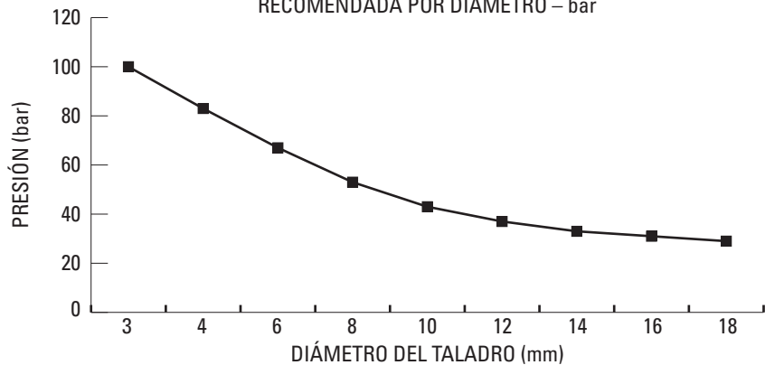
PRESIÓN DE REFRIGERANTE RECOMENDADA POR DIÁMETRO – bar
